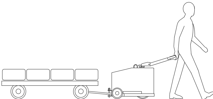
DTP053 型 けん引車 けん引容量 500 kg
