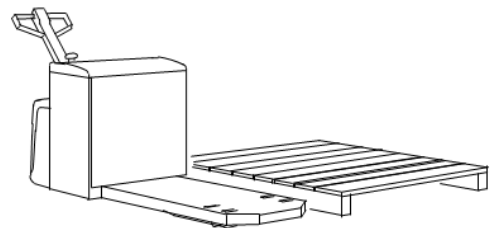
フォークをプラットフォーム型へ改造
